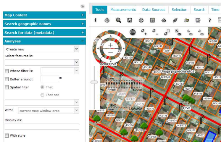
Slika 2 Kartica Analiza
