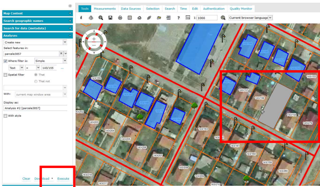
Slika 5 Rezultat pretrage
