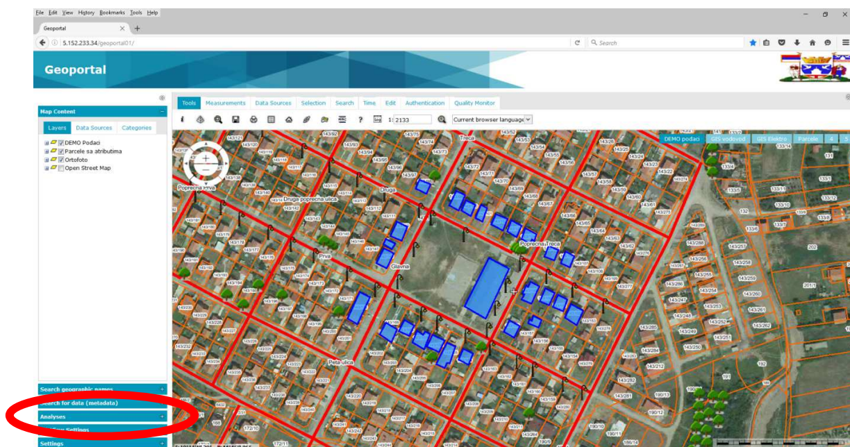
Slika 1 Početna stranica
